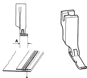
Piedino per applicazione cerniera sinistro Left zipper foot
