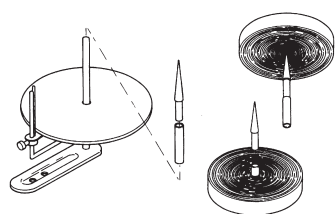
Portarotolo con cuscinetto a sfera e frenaggio Ball bearing - tension - tape rack
