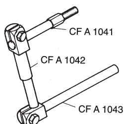
Attacco per Rimoldi - perno filettato 6 ma Bracket for Rimoldi - threaded pin 6 ma
