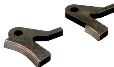
▶ Piedino per scarnitrice Spacing "feet", for skiving machine Regolatore di spessore durante la scarnitura 854 mm 50 361 mm 34 3616 mm 23 1486 mm 20
