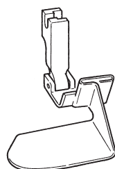
Piedino applicazione bande con guida limitatrice Lay-on foot with guide
