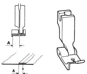
Piedino con guida fissa sinistra
