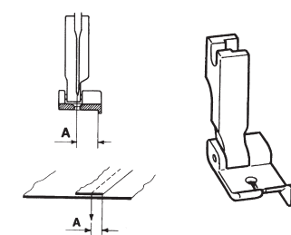
Piedino con guida fissa destra
