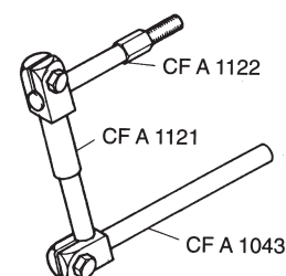
Attacco per PFAFF - perno filettato 5 ma Bracket for PFAFF - threaded pin 5 ma
