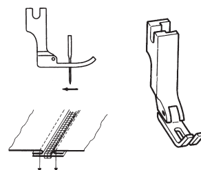
Piedino articolato per cerniere per machine a trasporto ago Hinged foot for zipper on needle feed machines
