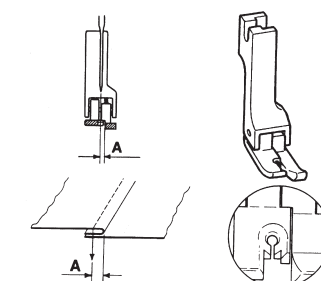
Piedino compensatore destro stretto per tessuti leggeri
