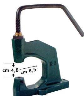
▼ Torchietto Manual press 463.3051 n. 2 Kg 2,800
