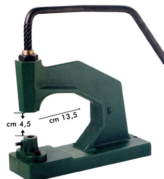
▼ Torchietto Manual press 463.3054 n. 5 Kg 5,500
