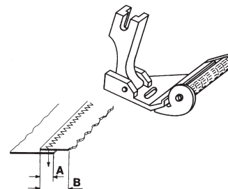
Piedino per applicazione pizzo Laces foot
