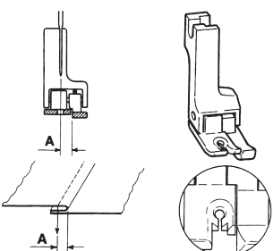
Piedino compensatore destro per tessuti leggeri
