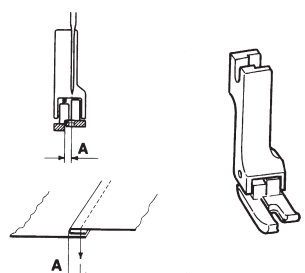
Piedino compensatore sinistro stretto
