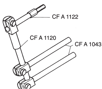
Attacco per PFAFF con due aste Bracket for PFAFF with two rods
