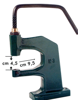
▼ Torchietto Manual press 463.3052 n. 3 Kg 3,200
