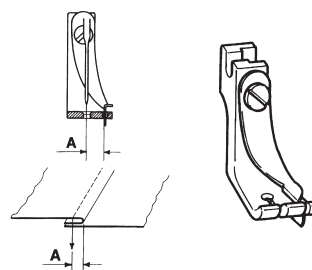
Piedino per ribattere con guida a molla Top stitching foot with spring guide
