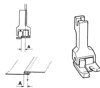
Piedino compensatore sinistro
